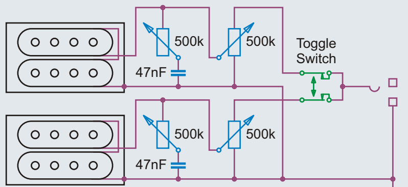
Schaltplan
