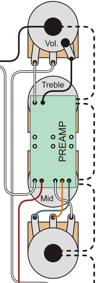
Masseverbindung über Kontrollblech
