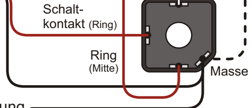
Stereo-Klinkenbuchse mit Schaltkontakt
